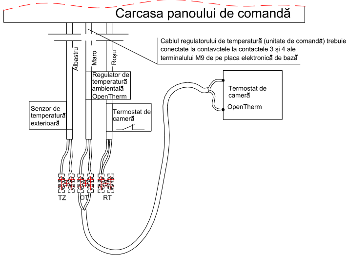
Img. 3.10.2 Conectarea regulatorului de temperatură OPENTHERM
