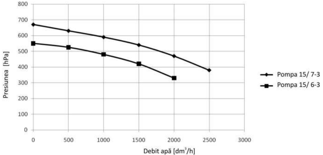
Img. 4.5.1 Caracteristica pompei
