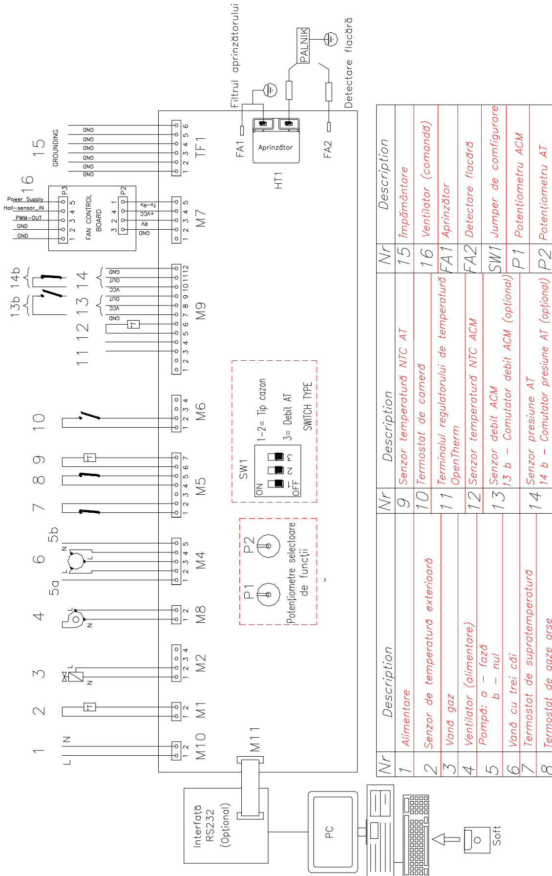
Img. 3.10.3. Schema de conexiuni electrice
