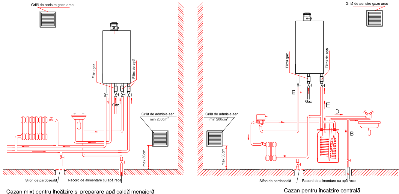
Img. 3.5.1. Cerințe pentru instalarea cazanului
