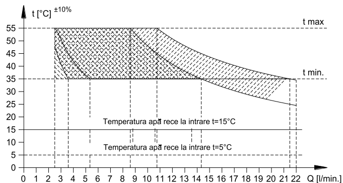
Img. 2.4.3.2. Temperatura ACM măsurată la racordul de ieșire din cazan în funcție de debit pentru tipul WINDSOR PLUS-30
