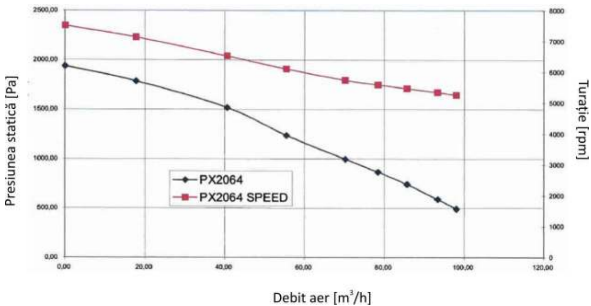
Img. 4.4.1 Caracteristica ventilatorului
