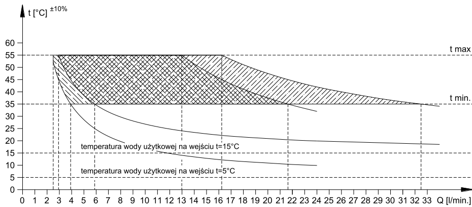
Img. 2.4.3.3. Temperatura ACM măsurată la racordul de ieșire din cazan în funcție de debit pentru tipul WINDSOR PLUS-50
