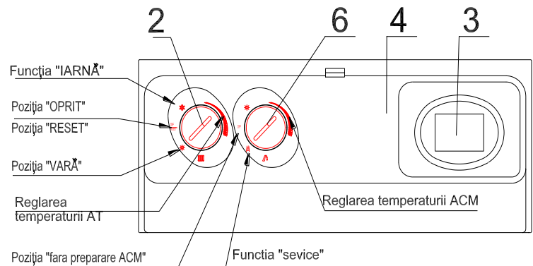
Img. 5.2.1. Panoul de comandă
