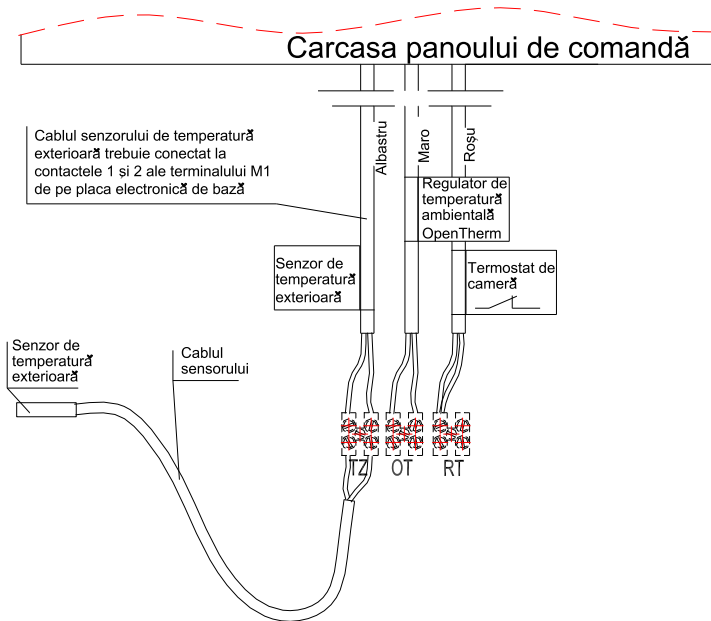
Img. 3.11.1 conectarea senzorului de temperatură exterioară
