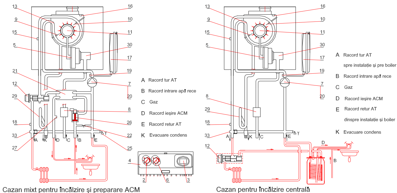
Img. 2.2.1.2. Diagrama de funcționare a cazanului
