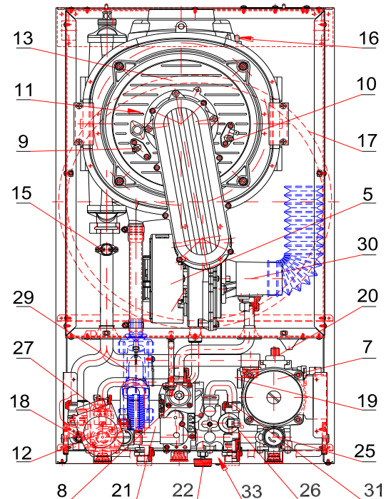
Img. 6.1.1.1 Interiorul cazanului
