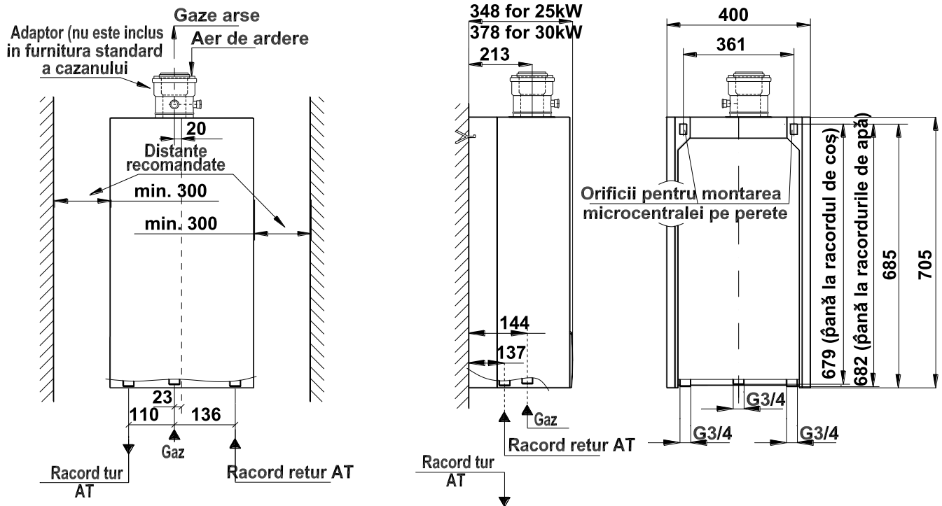
Img. 3.3.2. Dimensiuni de montare a cazanelor WINDSOR PLUS-25 și WINDSOR PLUS-30 pentru încălzire centrală
