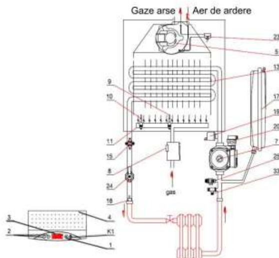
Fig. 2.2.1.2 Diagrama de funcționare a microcentralei
