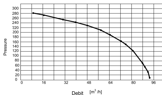
Caracteristica ventilatorului tip GOLD fig. 3000.08.00.00
