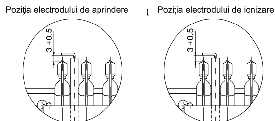
Fig. 6.1.2.1. Poziționarea electrozilor pe arzător
