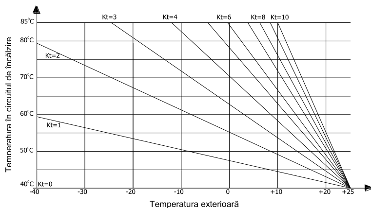
Fig. 2.4.1.1.1. Curba de încălzire
