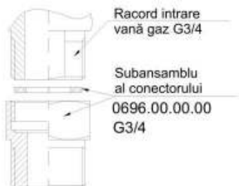
Fig. 3.4.1. Racordul de gaz
