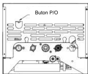
Vedere din partea inferioară a microcentralei
