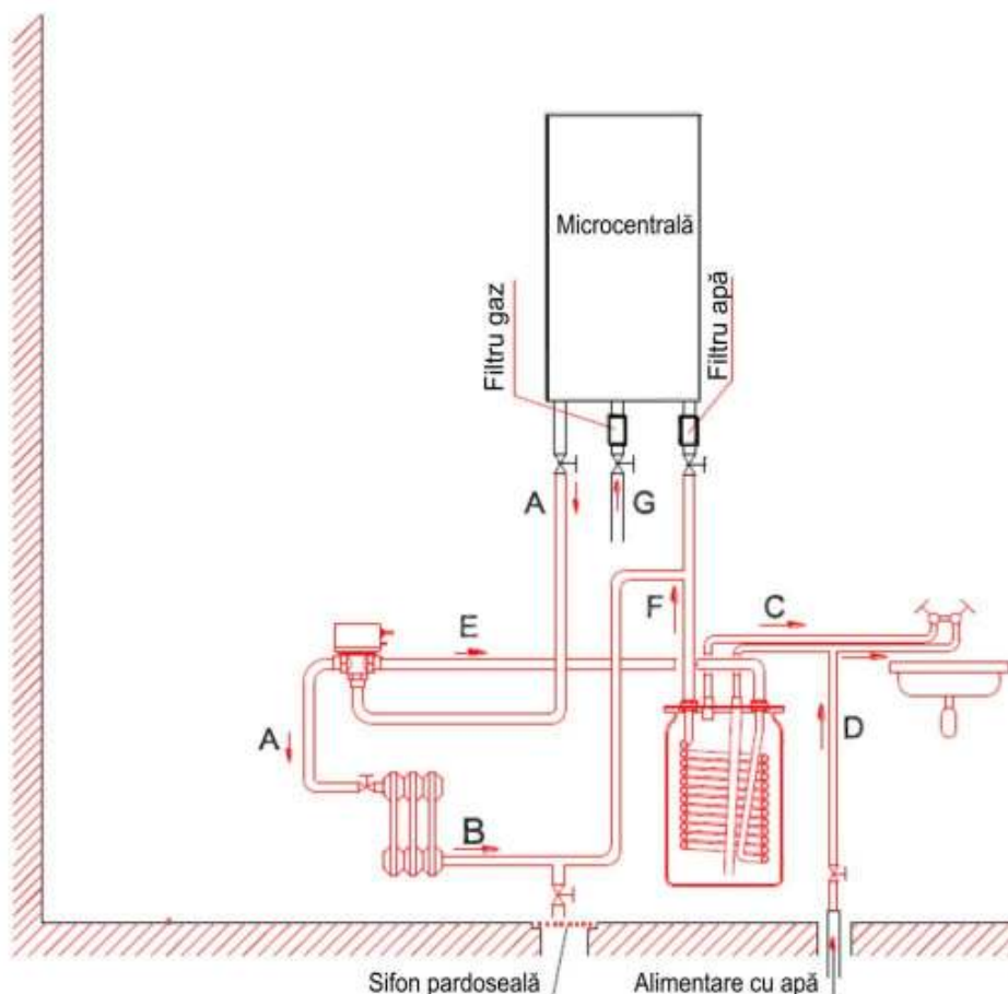
Fig.3.5.1 Cerințe pentru instalarea microcentralei
