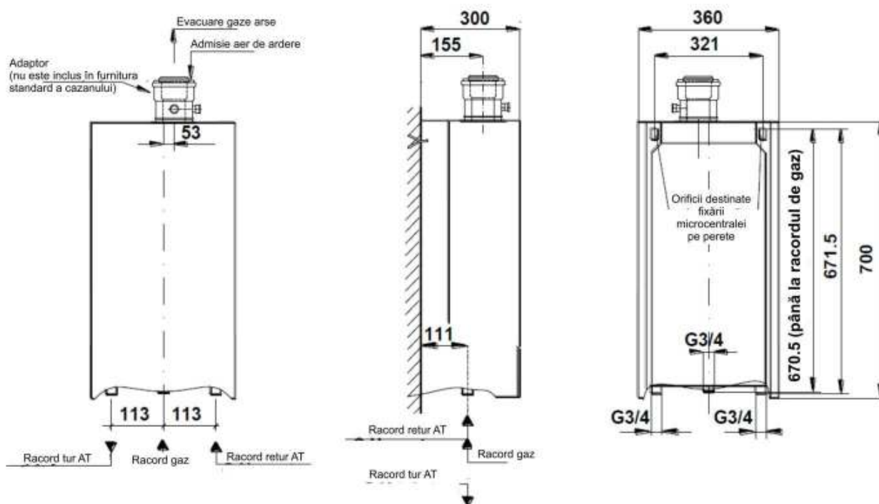
Fig. 3.3.1 Dimensiuni de instalare
